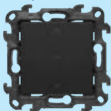
Przycisk roletowy pojedynczy trójpozycyjny (1-0-2) IP20/IP44, NZP1K.01/49 E17010104446
