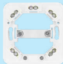
Gniazdo kuchenne do podłączania blatów płyt indukcyjnych i elektrycznych 5x2,5mm 2 GNK/5x4 biały E17020403620
