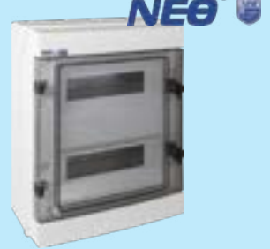
Rozdzielnica hermetyczna RH-24 IP65 500V AC 1000V DC 36.24 E20030000002
