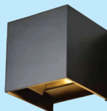
Oprawa elewacyjna 7W 360lm 4000K IP65 OE-10 antracyt E14040202388
