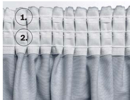
Fot. 6 Jeśli zaczepisz haczyk o górną „kieszonkę” (1) - dodaj 2 cm, a jeśli o dolną (2) - dodaj 5 cm do wysokości zasłony.
