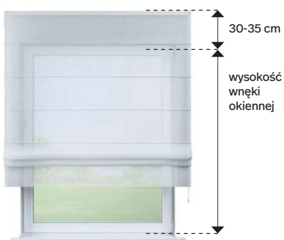
Montaż do ściany roleta Padva
