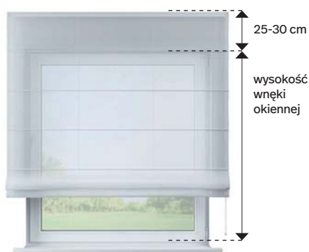
Montaż do ściany roleta Capri
