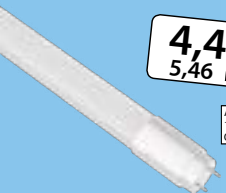
F Świetłówką LED 18W 1850lm 6500K 120 cm EK8244 E24120002911
